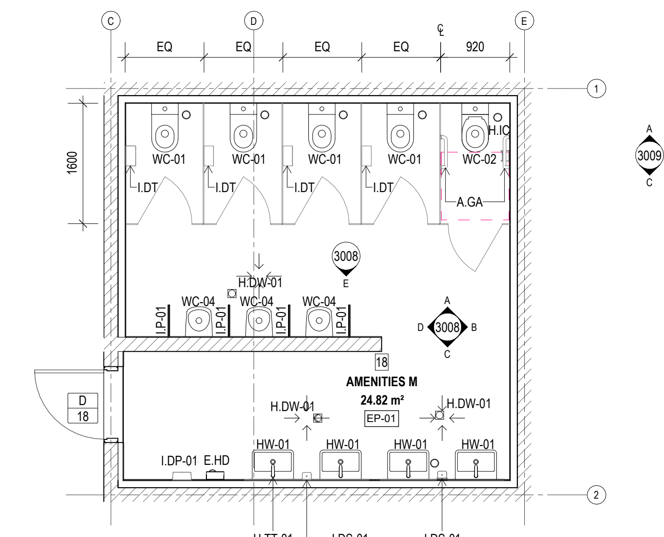
1 PLAN AMENITIES M Scale: 1:50
