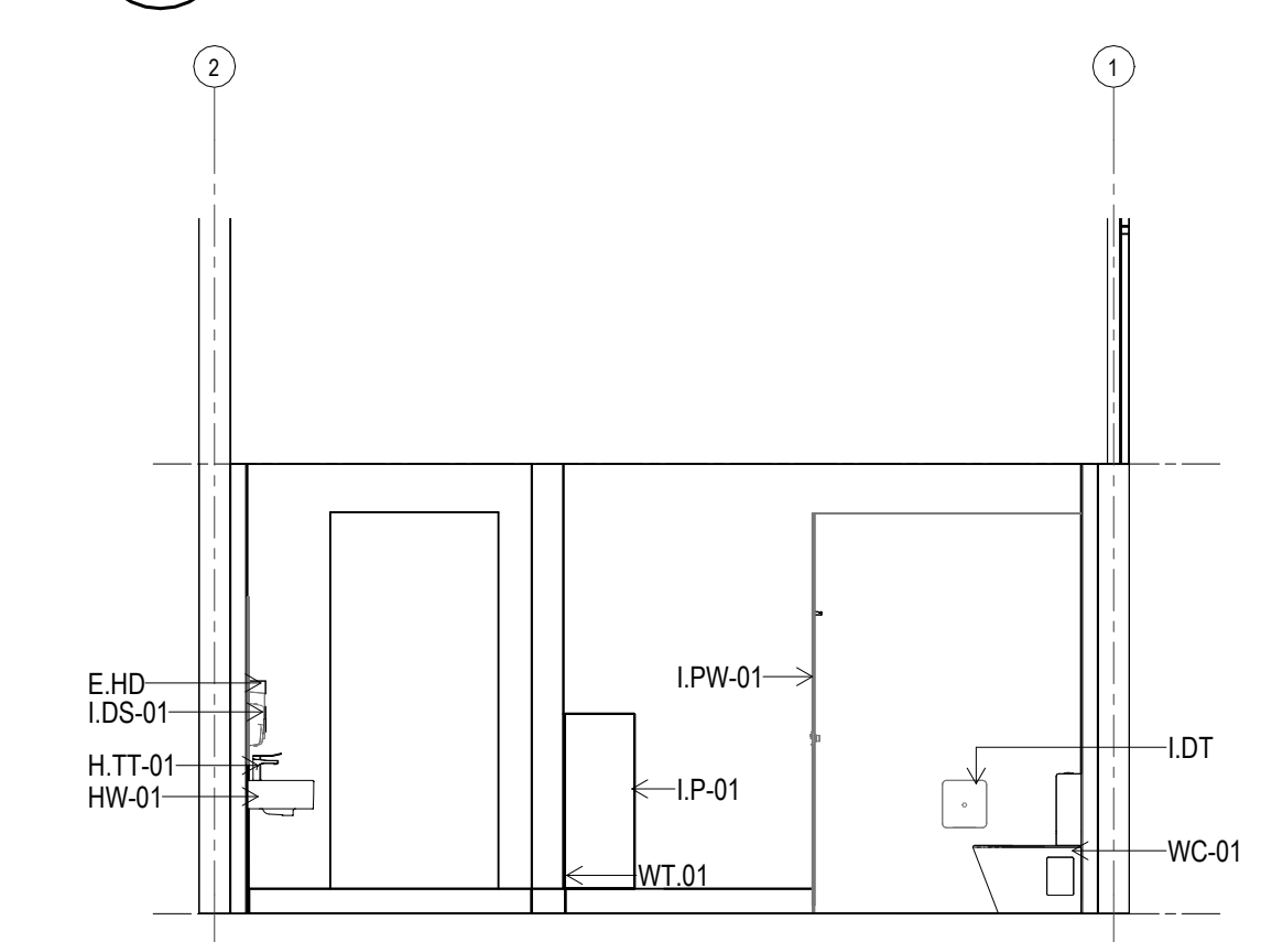
D ELEVATION AMENITIES M Scale: 1:50
