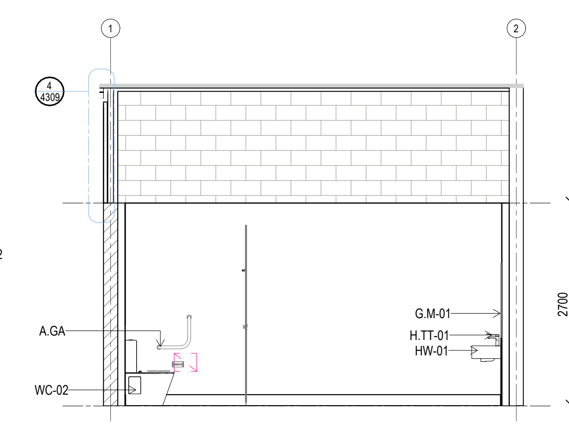
B ELEVATION AMENITIES M Scale: 1:50
