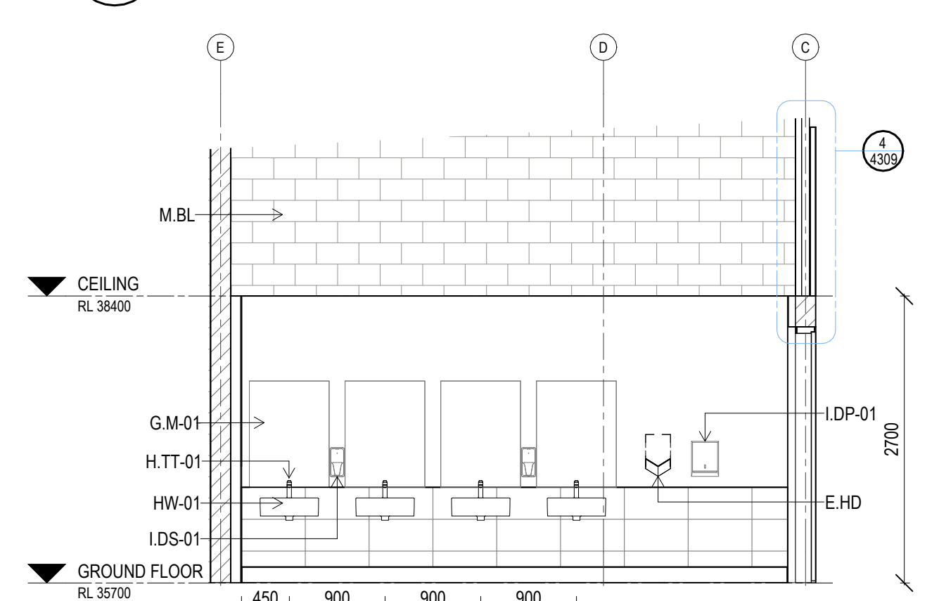
C ELEVATION AMENITIES M Scale: 1:50
