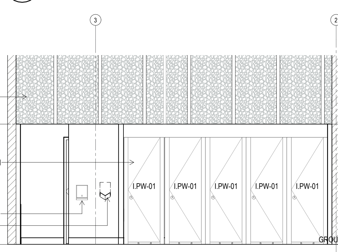
J ELEVATION AMENITIES F Scale: 1:50
