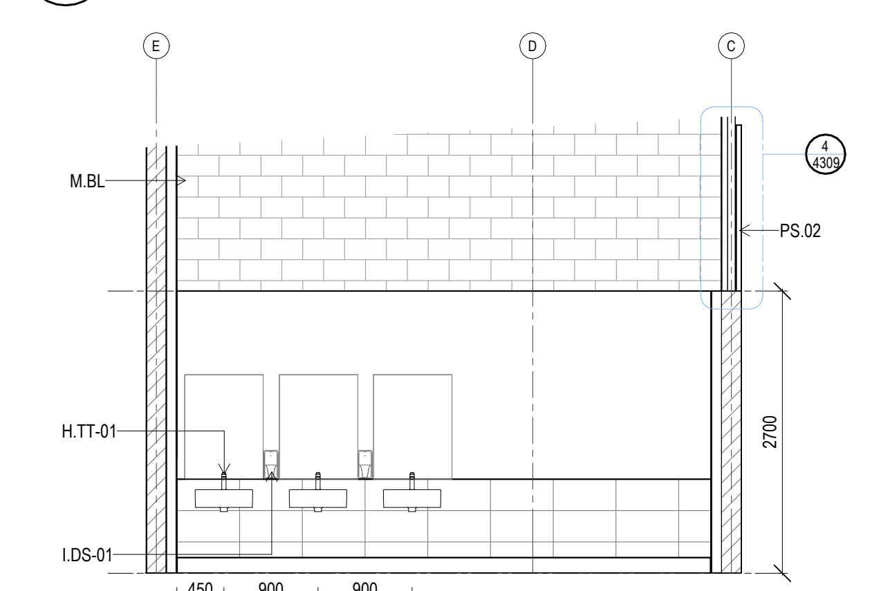
H ELEVATION AMENITIES F Scale: 1:50
