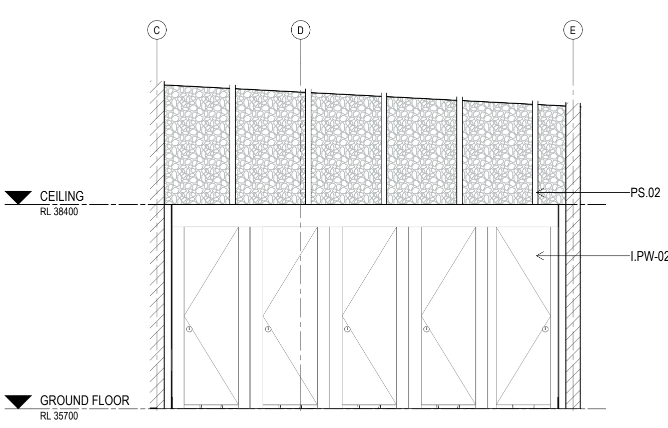
A ELEVATION AMENITIES M Scale: 1:50
