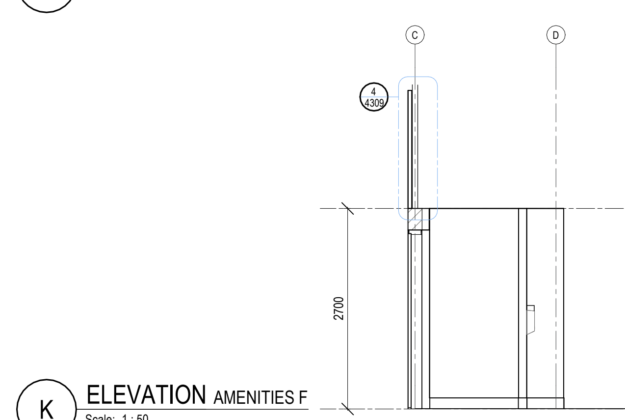
K ELEVATION AMENITIES F Scale: 1:50
