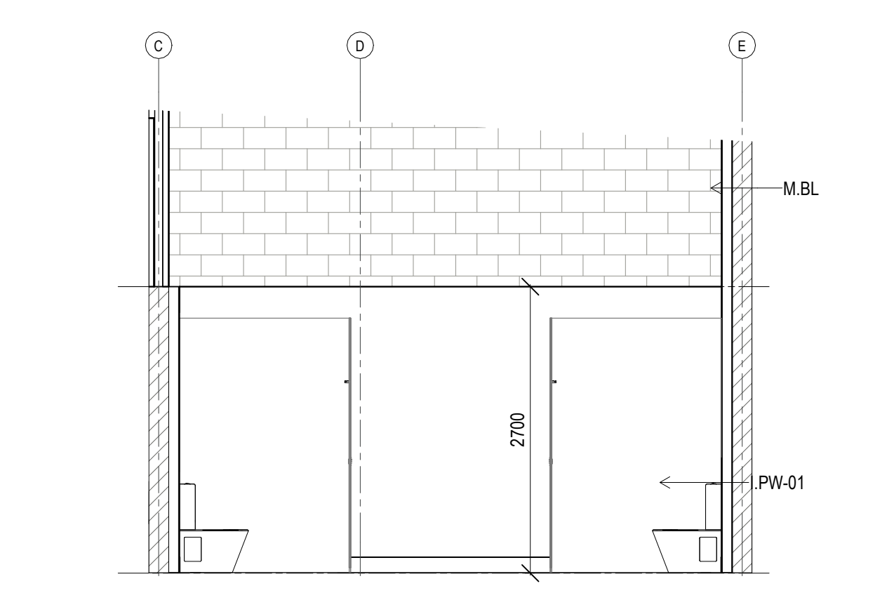
F ELEVATION AMENITIES F Scale: 1:50
