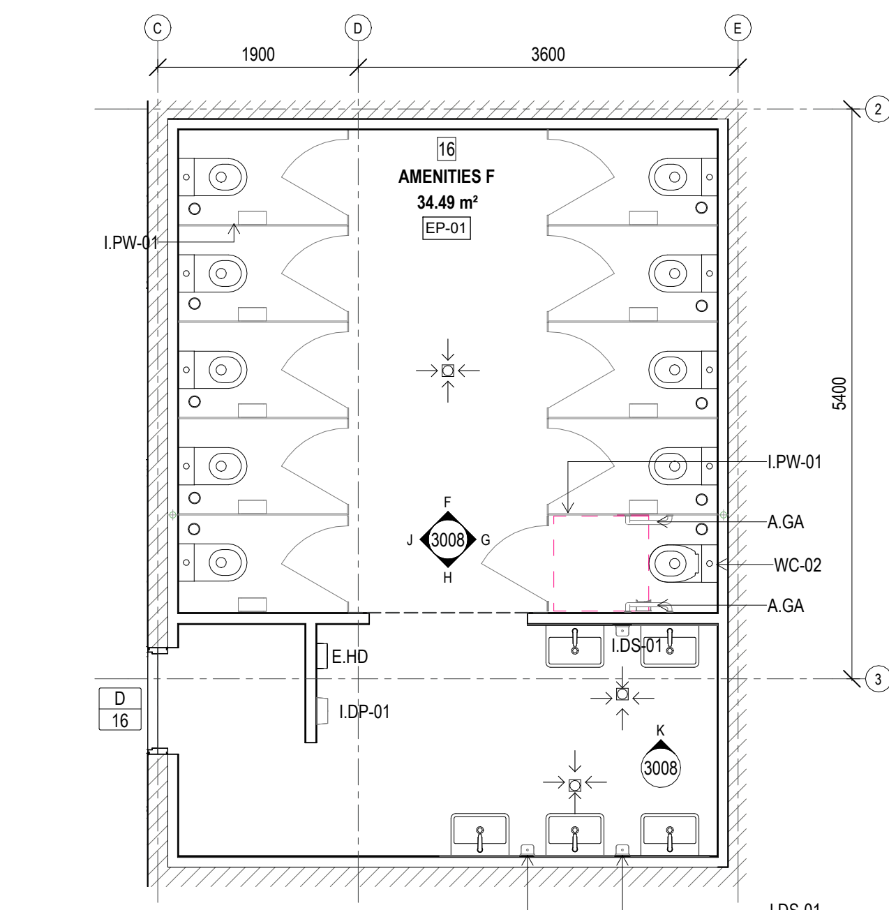
3 PLAN AMENITIES F Scale: 1:50
